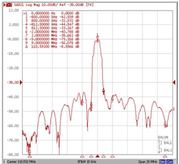
Attenuation
