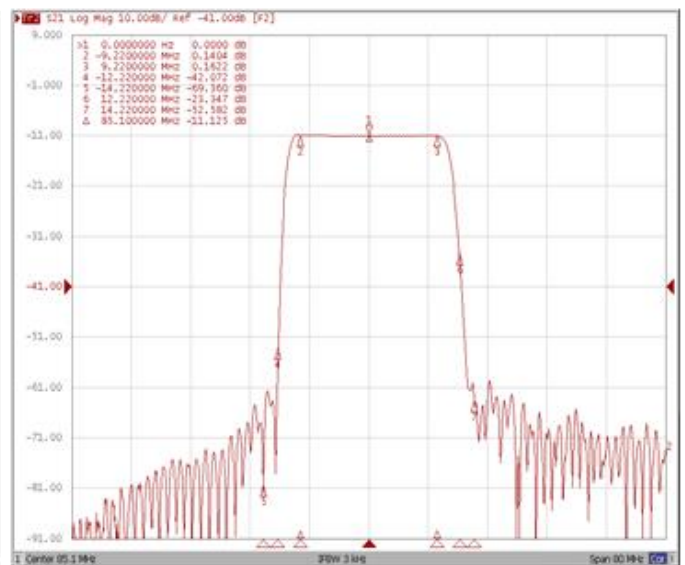
Attenuation
