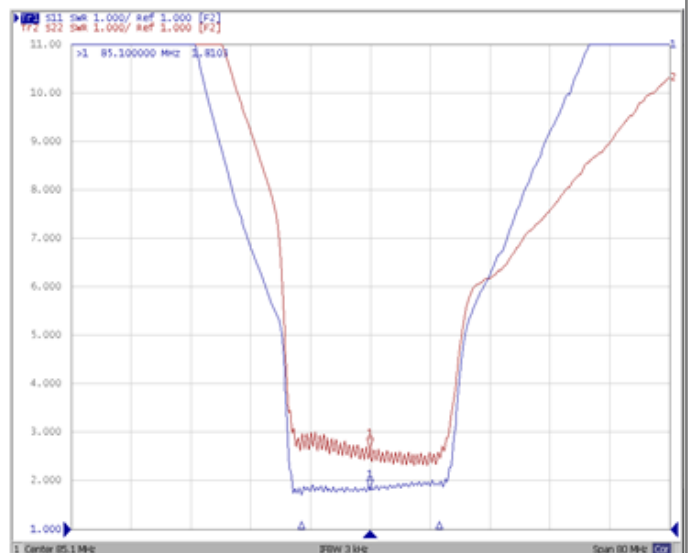
VSWR
