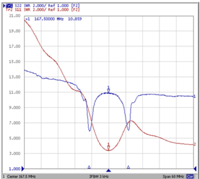
VSWR
