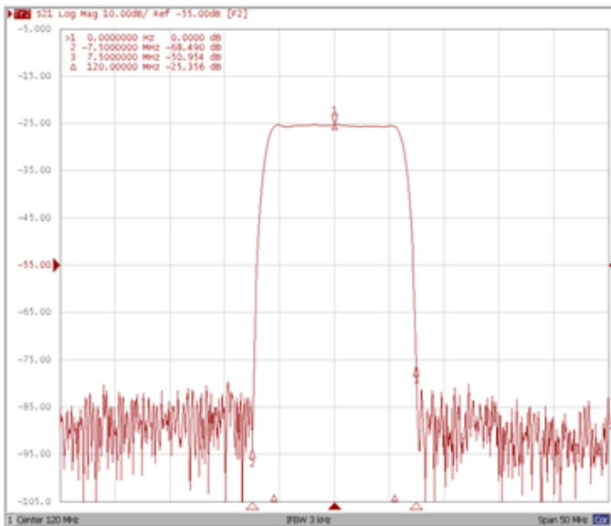
Attenuation Fo±7.5MHz
