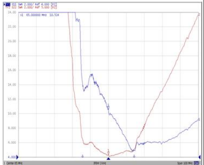
VSWR
